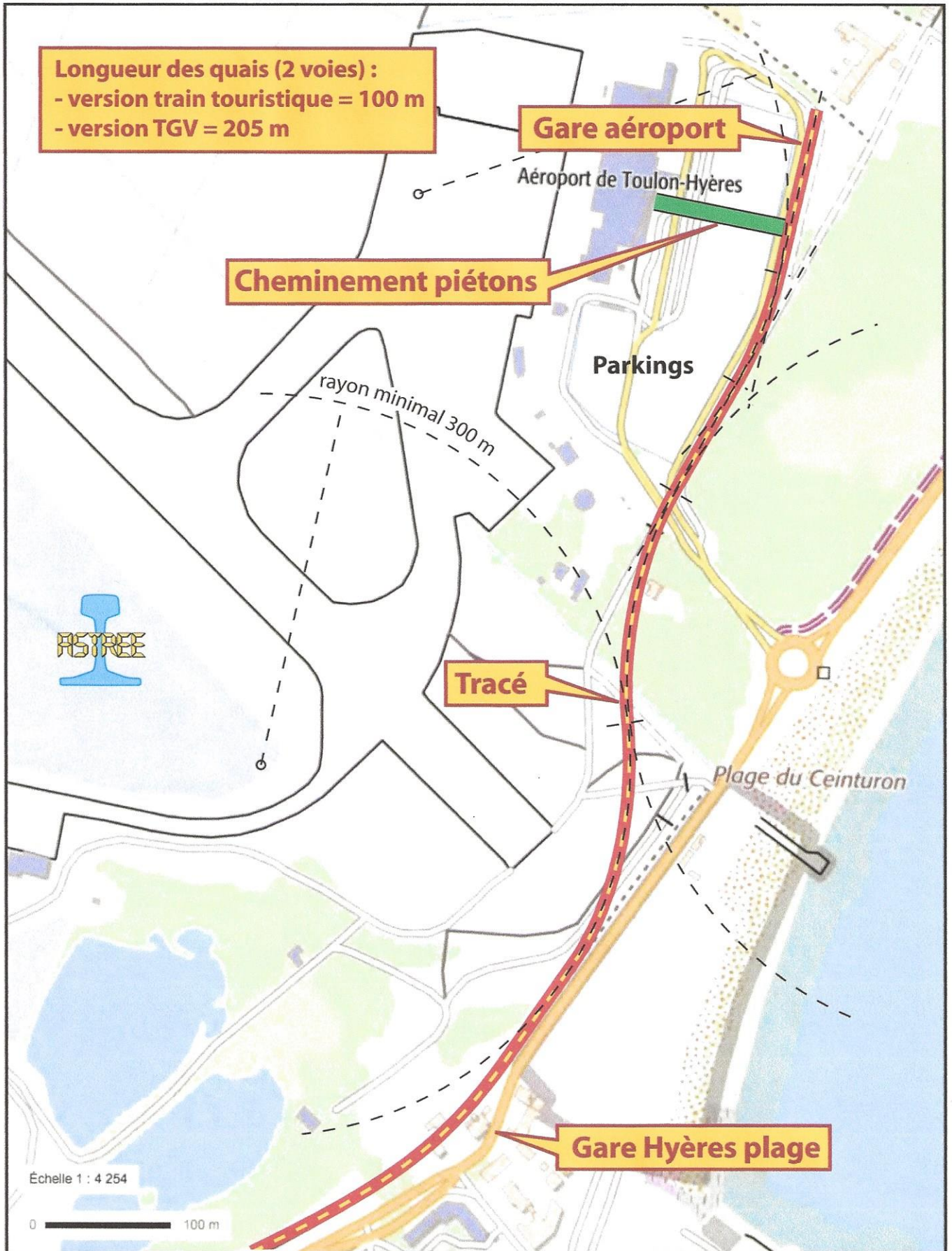
Tracé de la liaison entre la gare de Hyères-Plage et l'Aéroport Rayon minimal des courbes = 300 m
